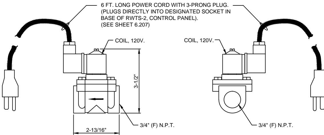
END ELEVATION
